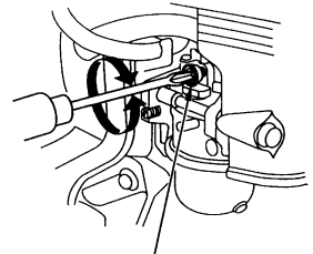
GASHEBELANSCHLAGSCHRAUBE
