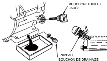
Moteur Honda/Robin
